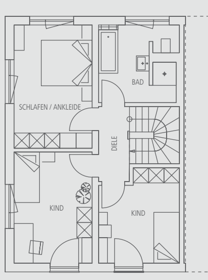
Obergeschoss, ca. 52 m 2 NGF.
